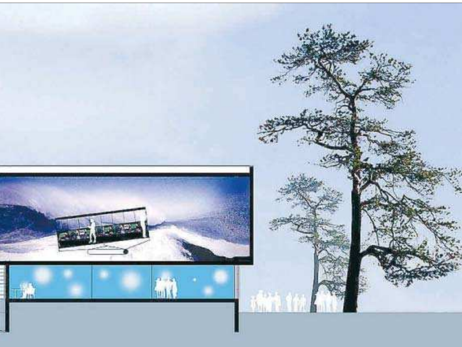
lаторer. Här ett snitt genom byggnaden sett från söder mot norr. Snittet går tvärs genom byggnaden i öst-västlig riktning. Foto: ARKITEKTBYRÅ MARKUS LINDROOS KB
