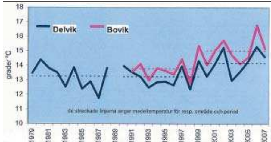
Vattentemperatur. Vattnet runt Åland har blivit varmare under de 30 senaste åren. Mätningarna har gjorts utanför Delvik i sund och i Hammarland Bovik.
