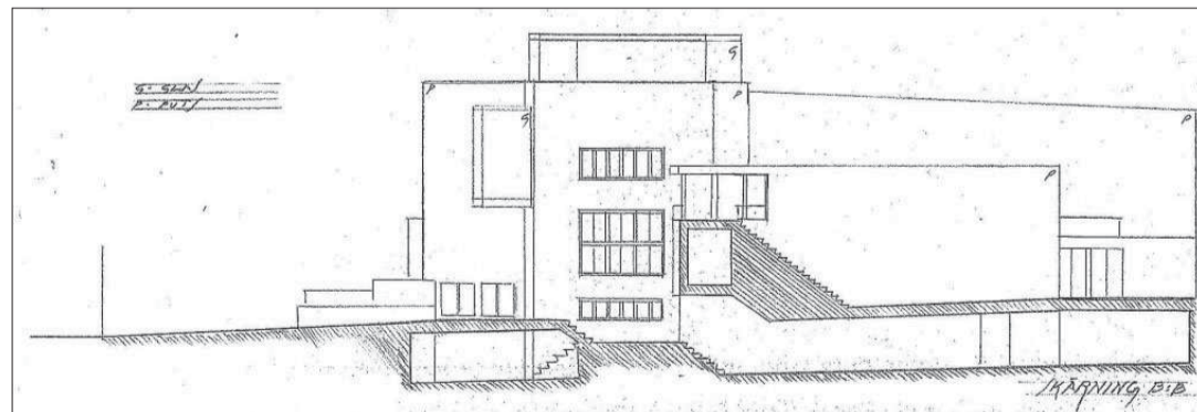
Fasad. Fasaden mot öster med utbyggnaden för den nya salongen. Påbyggnaden på tredje våningen har också dragits in för att ge rum för en terrass.
